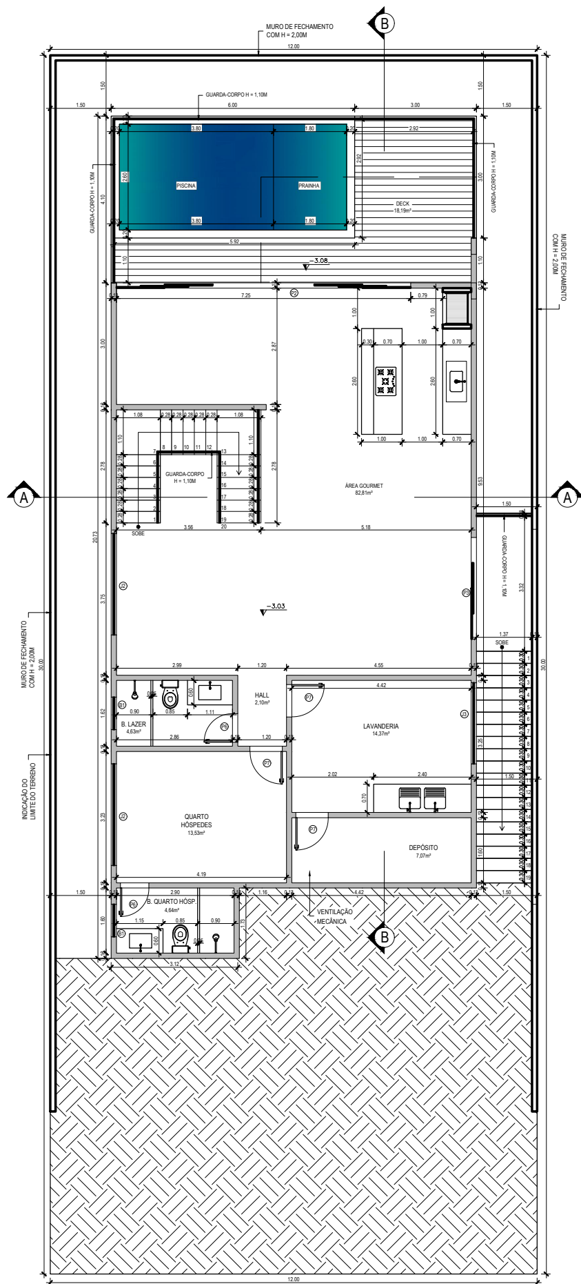
PLANTA BAIXA SUB-SOLO ESCALA 1/50
